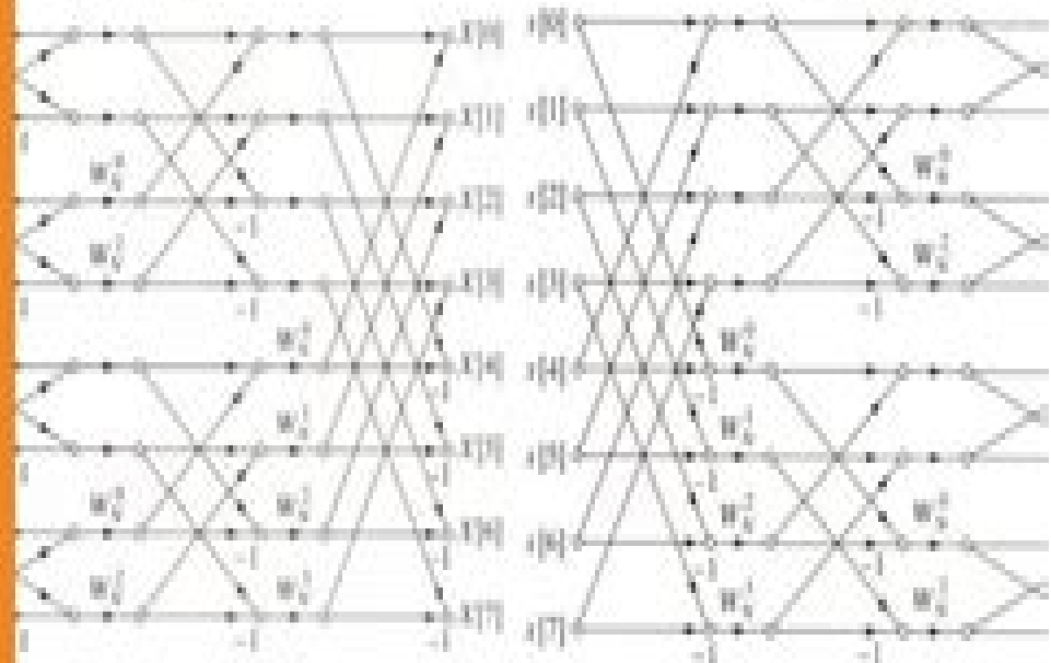
DIF FFT
