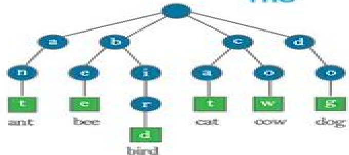
Trie
