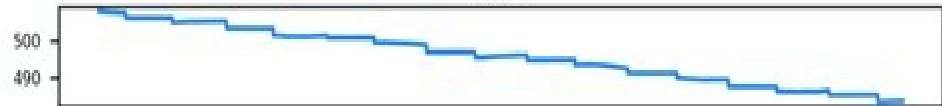
Trend
